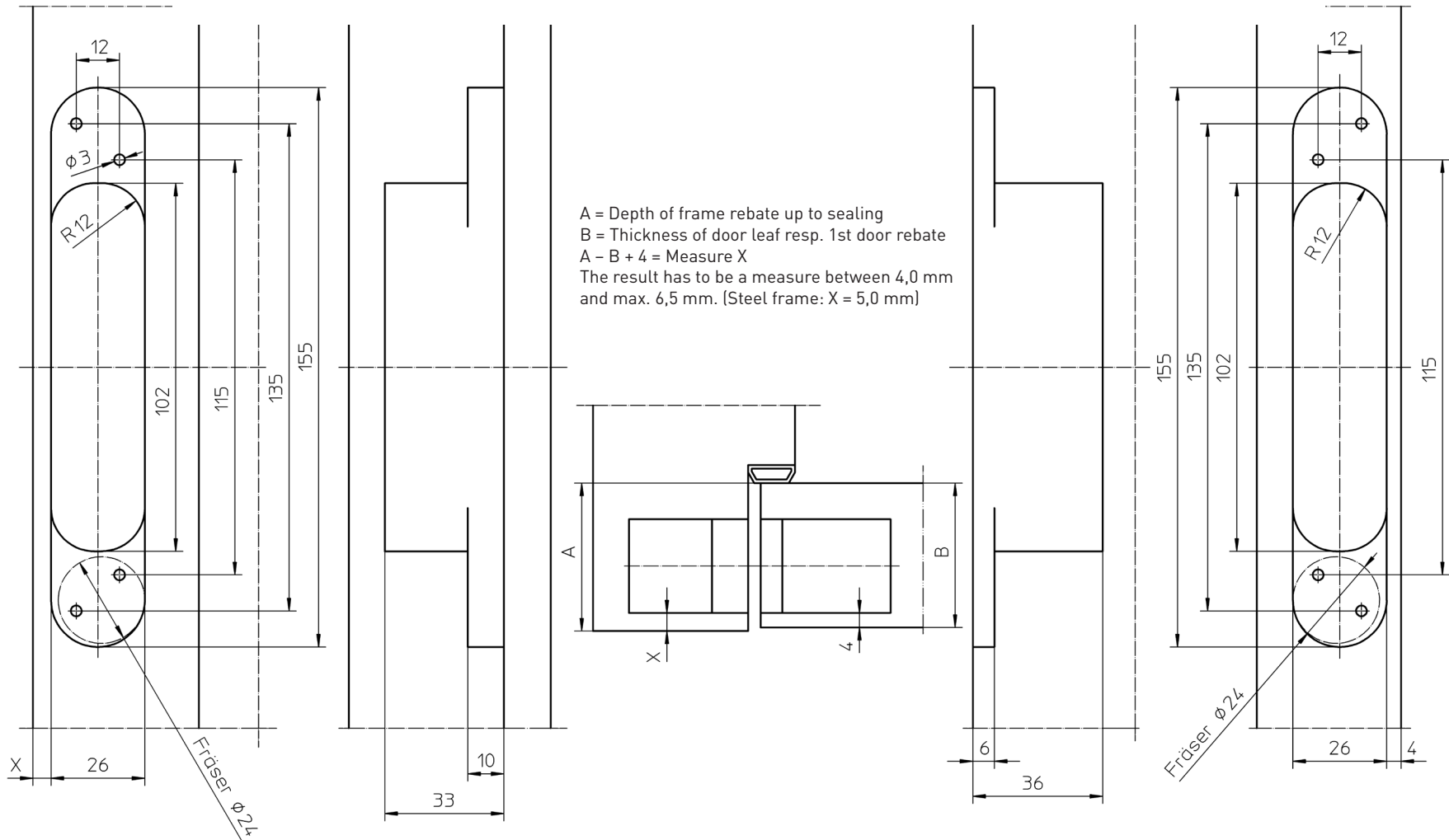
MILLING : DOOR LEAF
